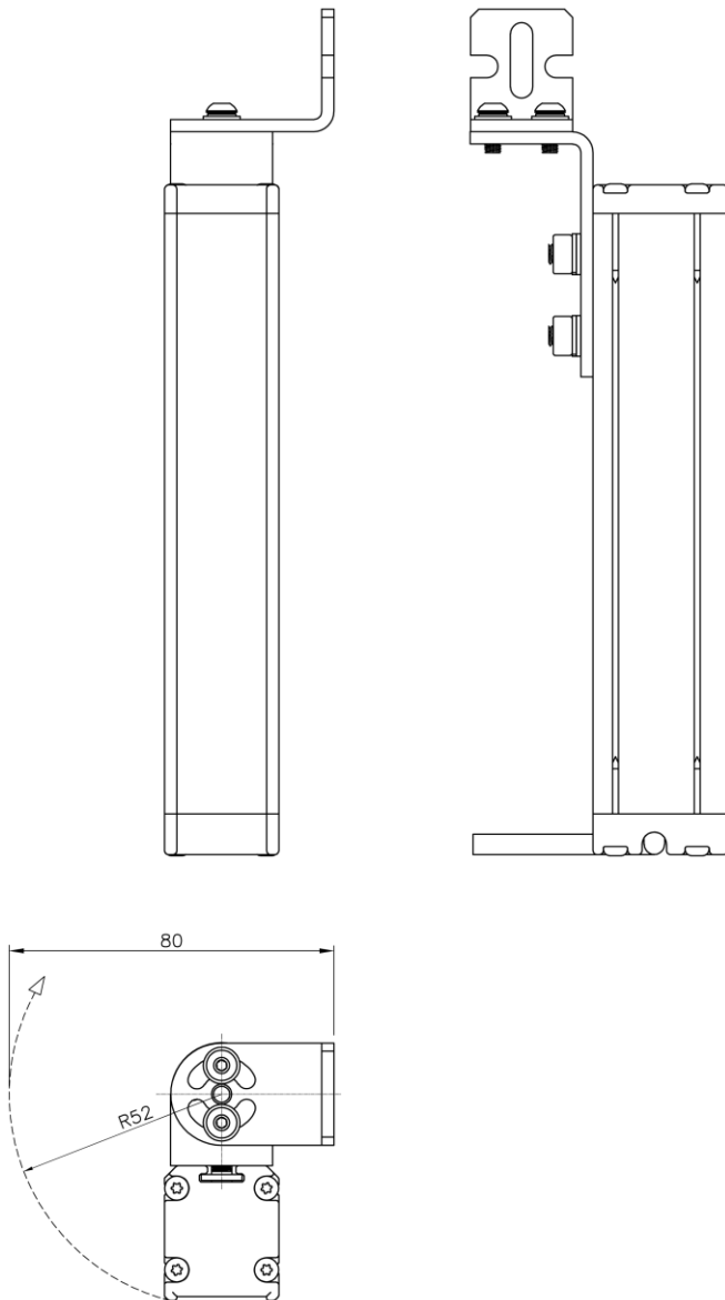
MONTAGGIO SCORREVOLE / SLIDING ASSEMBLY
