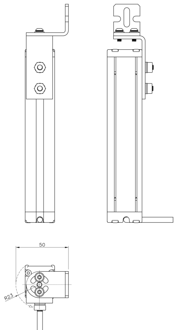
MONTAGGIO CON CORSA RIDOTTA / ASSEMBLY WITH REDUCED STROKE
